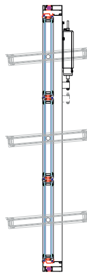
Ouverture/Fermeture pneumatique
