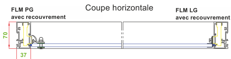
Coupe horizontale double vantelle
