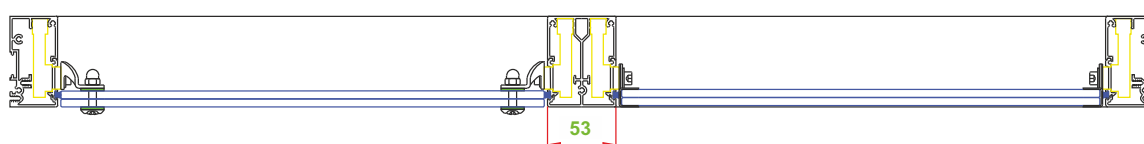
Coupe horizontale double vantelle
