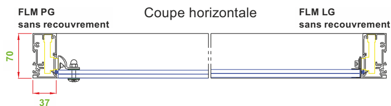
Coupe horizontale double vantelle
